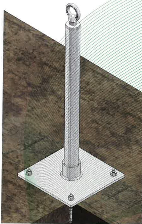
Bild 1: Anschlageinrichtung Typ: LUX-top® Abseilpunkt (Montagebeispiel)
