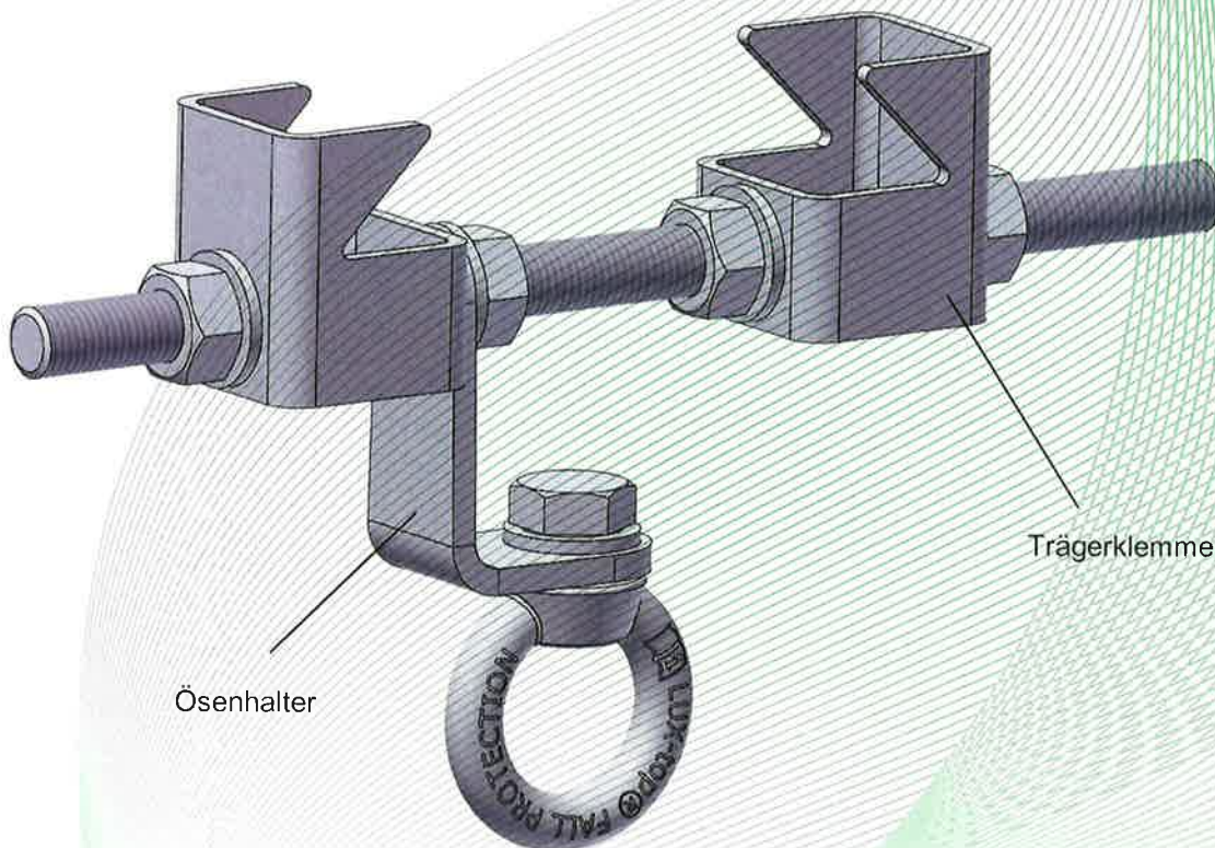
Bild 1: Anschlageinrichtung, Typ: LUX-top® QUICKFIX II
